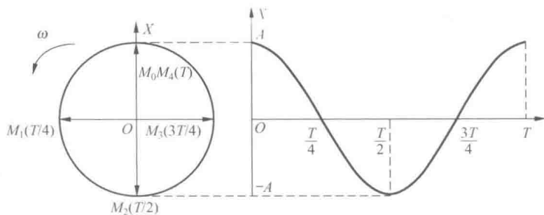
图 11-7 旋转矢量图和简谐振动的 x-t 图
