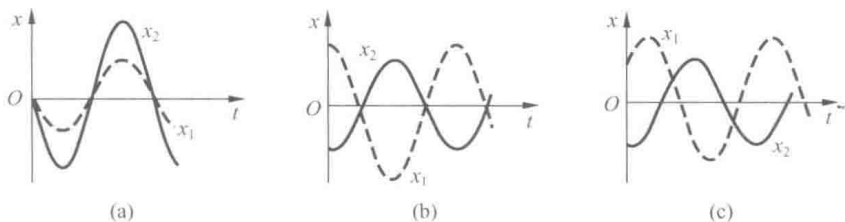
图 11-3 相位差的图示法
