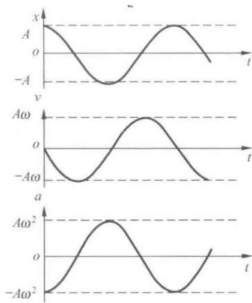
图 11-2 简谐振动的 x-t 图、 v-t 图与 a-t 图
