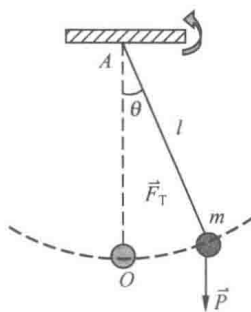
图 11-13 单摆
