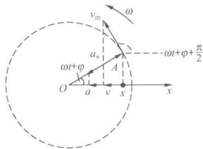
图 11-8 旋转矢量图中的速度和加速度
