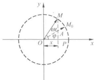
图 11-6 旋转矢量图
