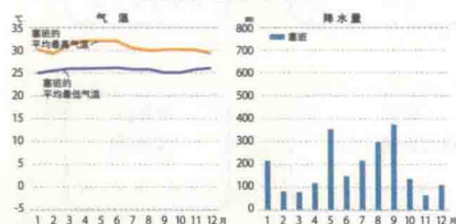
塞班的气温和降水量
