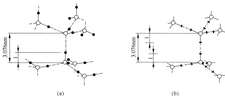
图 1-3 冰结构中氢原子的位置
