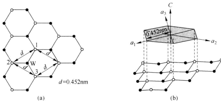
图 1-1 冰的基础平面（圆圈代表水分子的氧原子，空心和实心圆圈分别表示上层和下层的氧原子）
