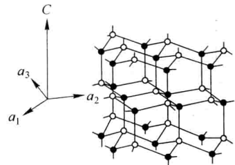
图 1-2 冰的扩展结构
