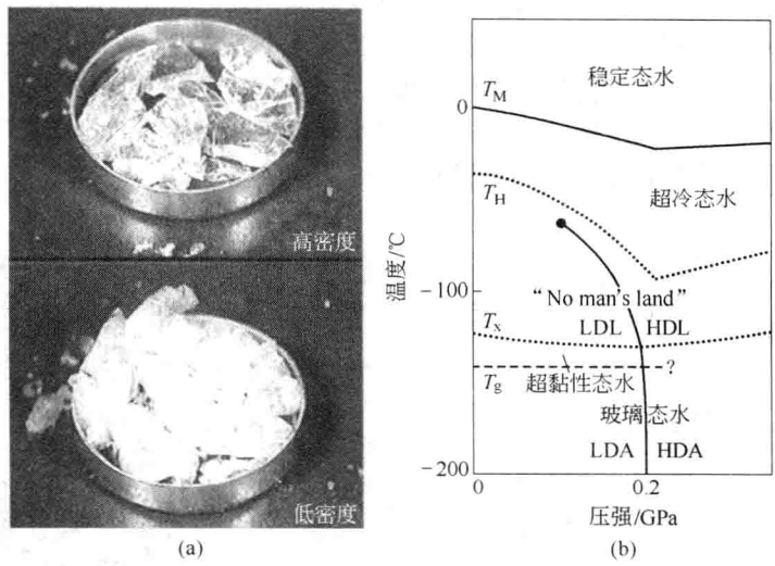
图 1-5 两种玻璃态水和预测的液-液相变的相关相图
