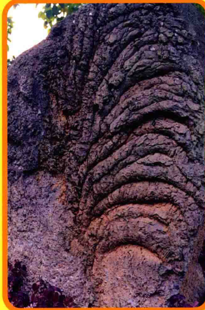
绳状玄武石
