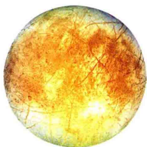
木星的卫星木卫二
