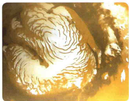
火星两极的冰盖
