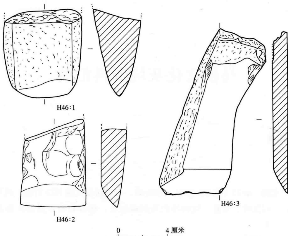
图 f1-0-1B 马桥文化 H46 出土器物
