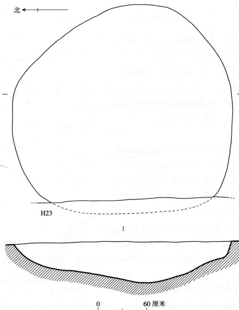
图 f1-0-1A 马桥文化 H46 平剖图
