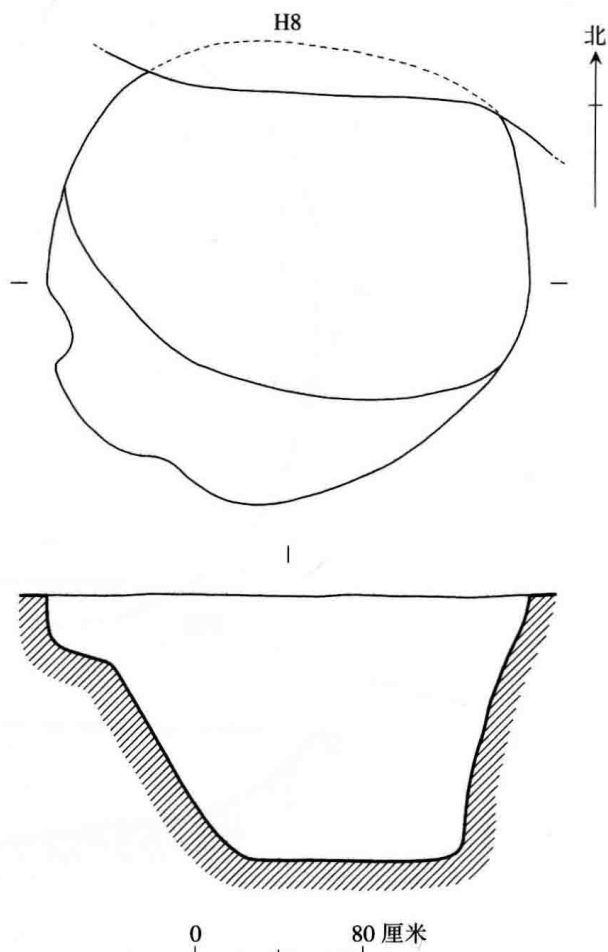
图 f1-0-2A 马桥文化 H94 平剖图
