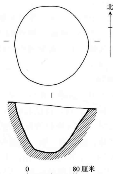
图 f1-0-4A 马桥文化 H213 平剖图
