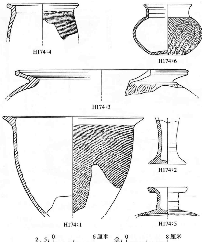
图 f1-0-3B 马桥文化 H174 出土器物
