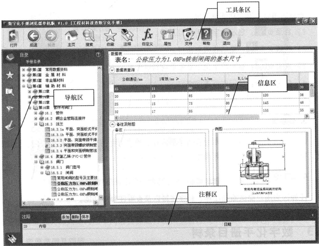
图 2-2 数字化手册主窗口
