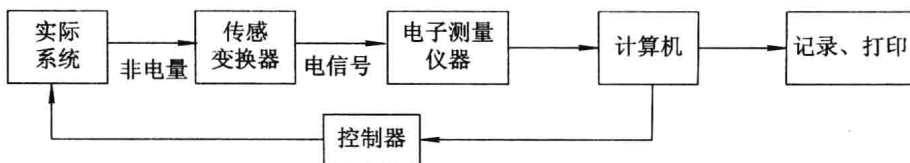
图 1.1-1 自动过程控制系统中非电量的测量
