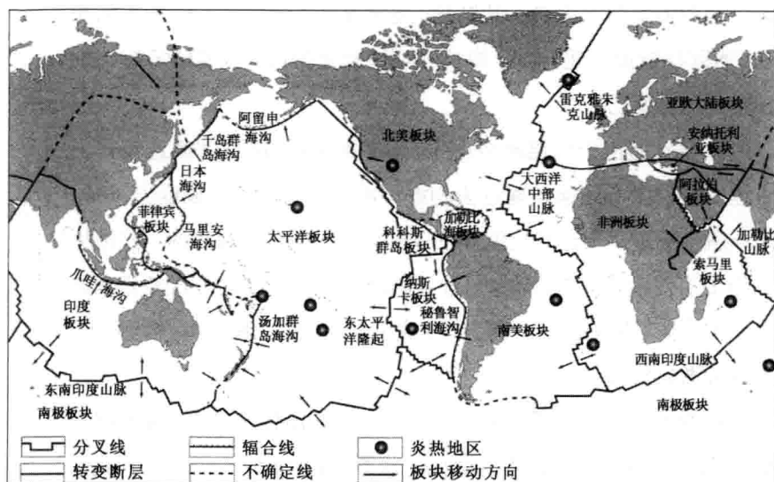
图1 大陆板块构造
