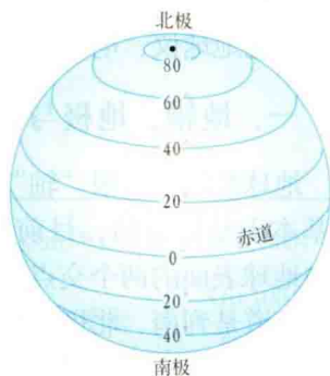
图1.7 纬线、纬度
