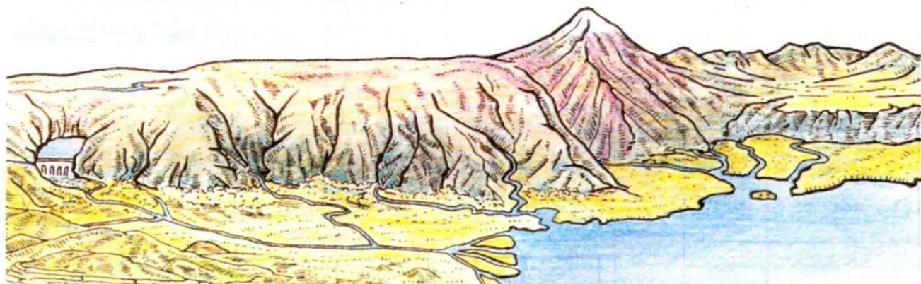
图1.17 地形素描图
