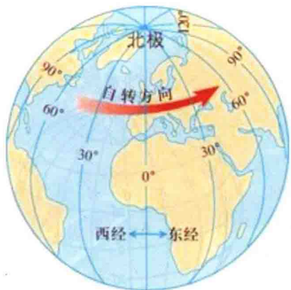
图1.5 经线与经度
