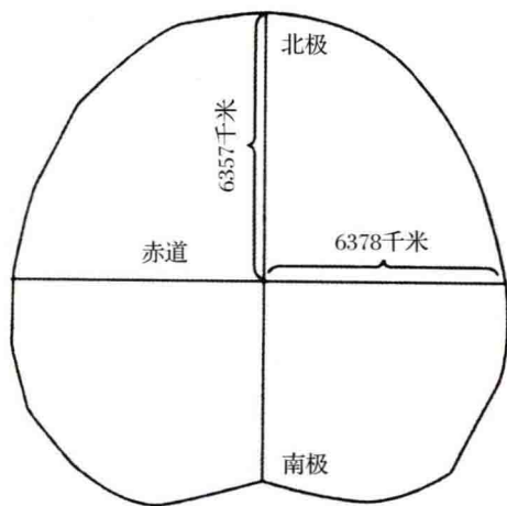
图1.1 地球的形状
