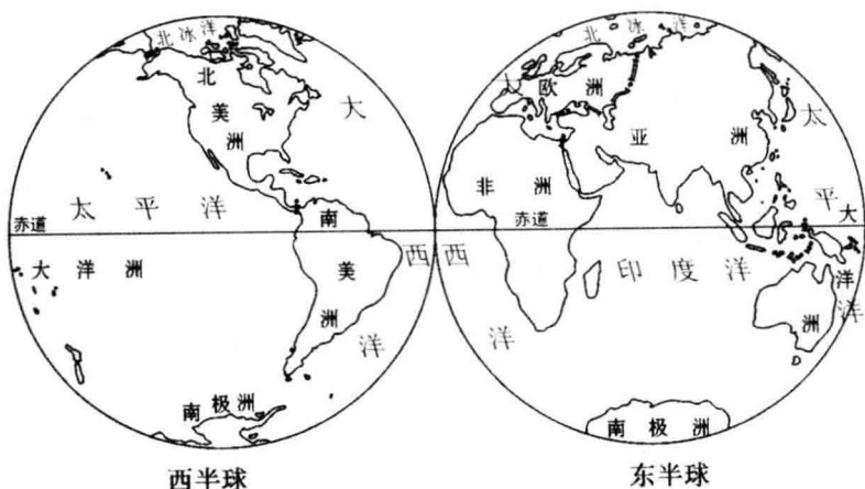
图1.6 东、西半球
