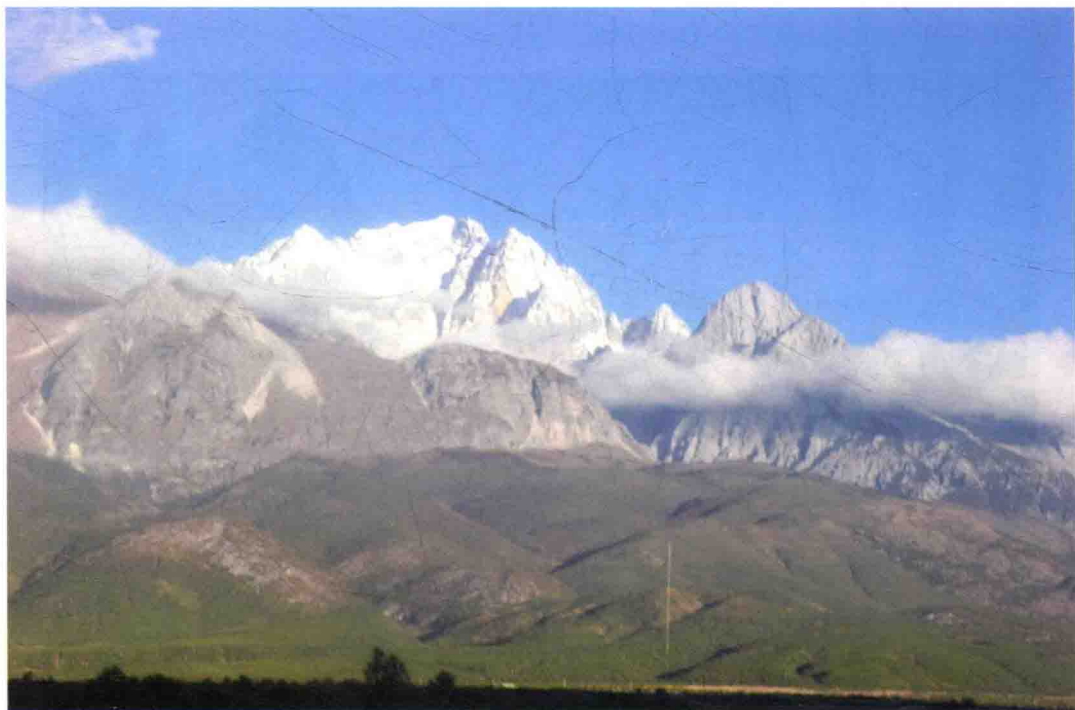
云南丽江玉龙雪山
