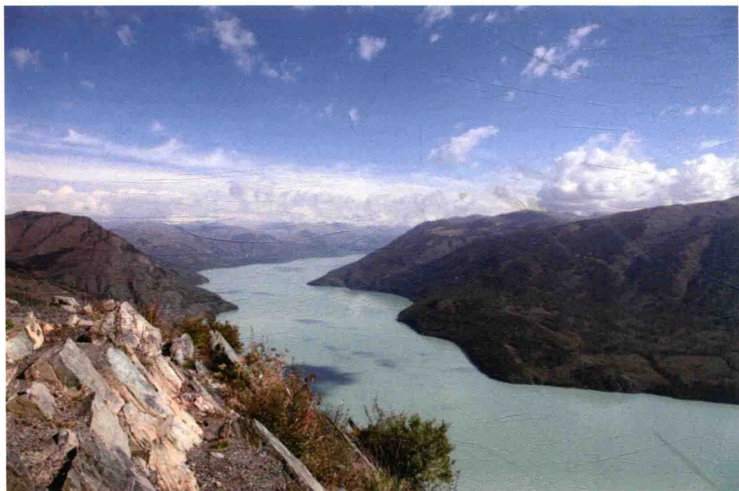
新疆噶纳斯地质景观
