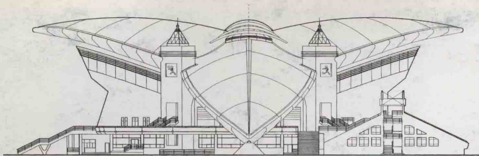
南立面
