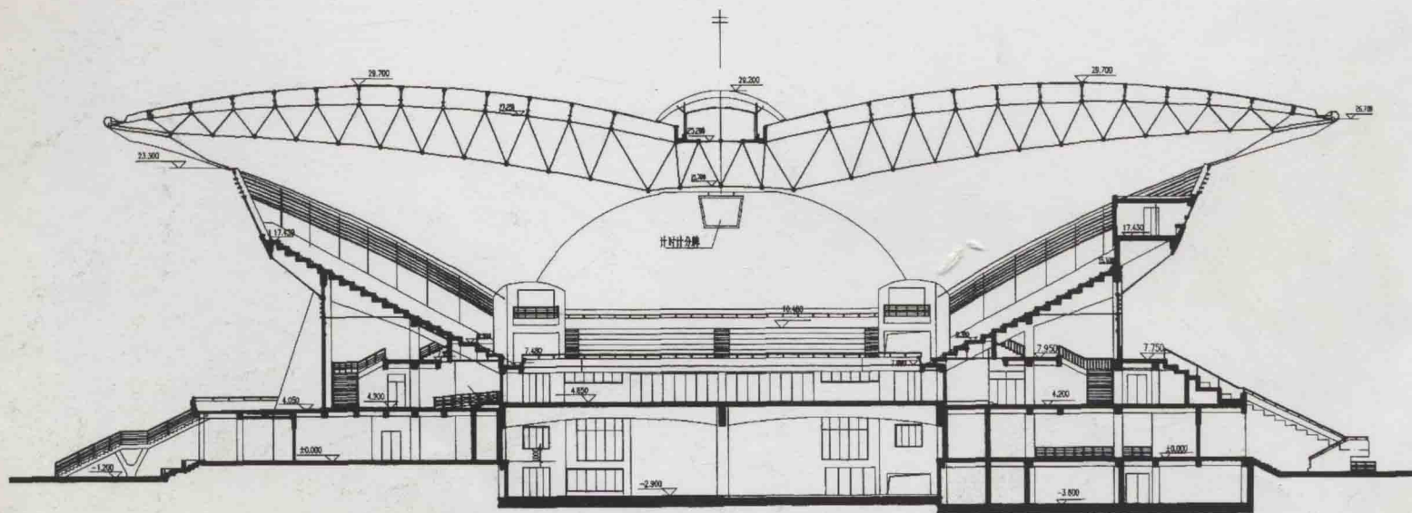
1-1 剖面
