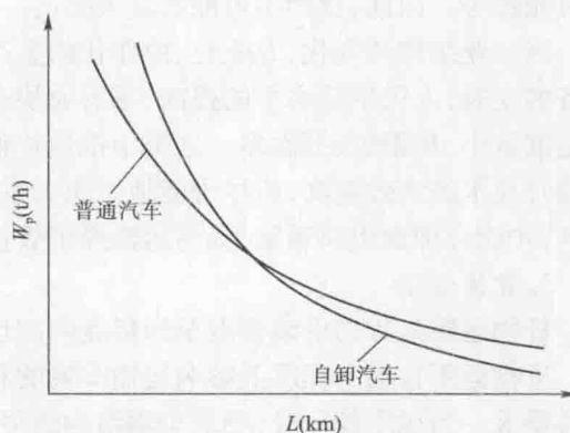
图 1-5 不同车辆(普通汽车与自卸汽车)运输生产率 W_p 的比较
