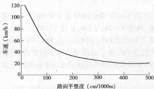
图 1-1 汽车允许速度和路面不平度的关系
