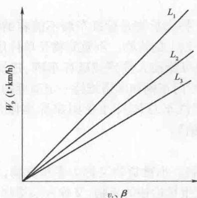
图 1-2 汽车运输生产率 W_p 与汽车技术速度 v_t 和行程利用率 \beta 的关系 ( L 为货物运距, 且 L_1 < L_2 < L_3 )
