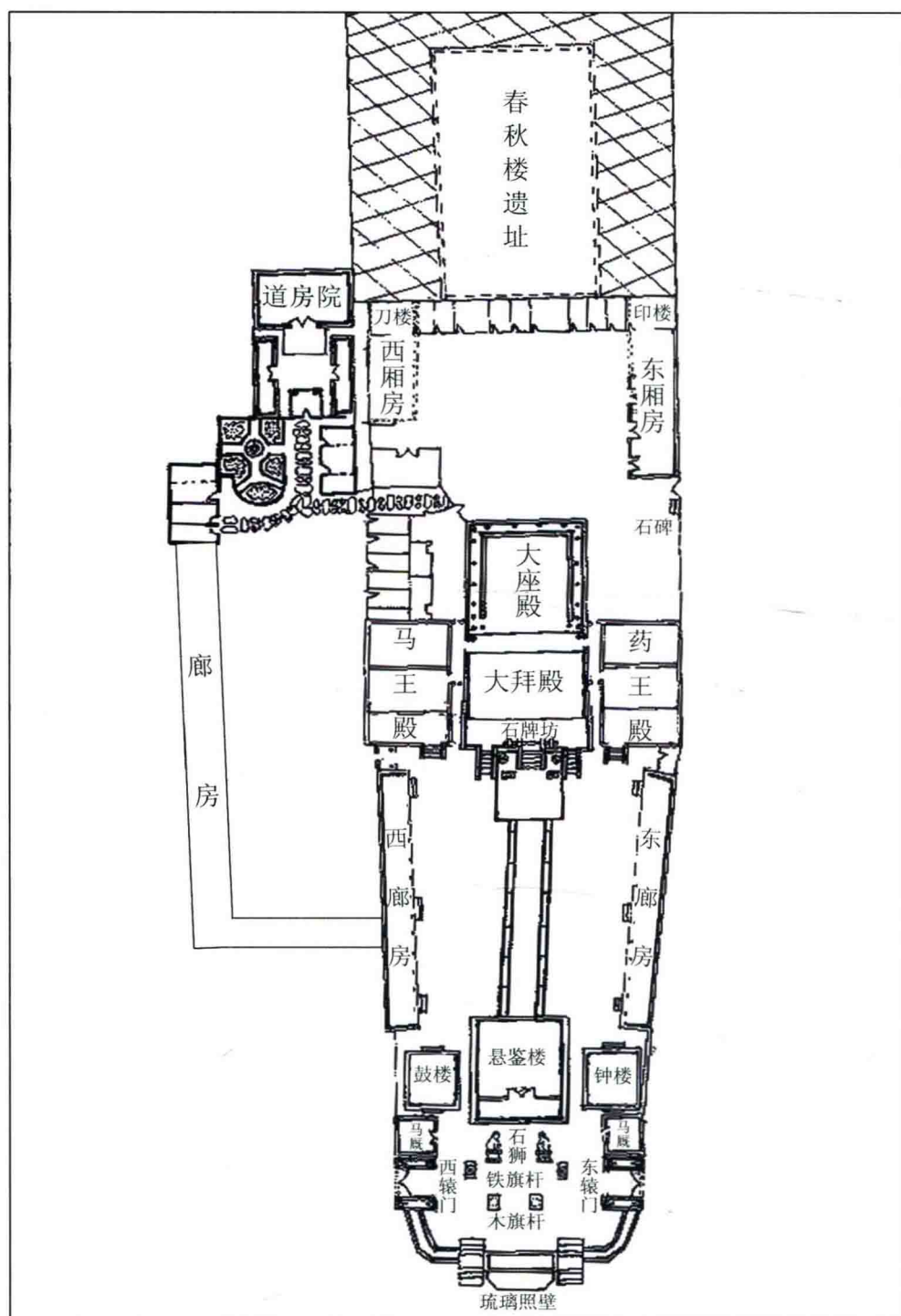
社旗山陕会馆平面图
