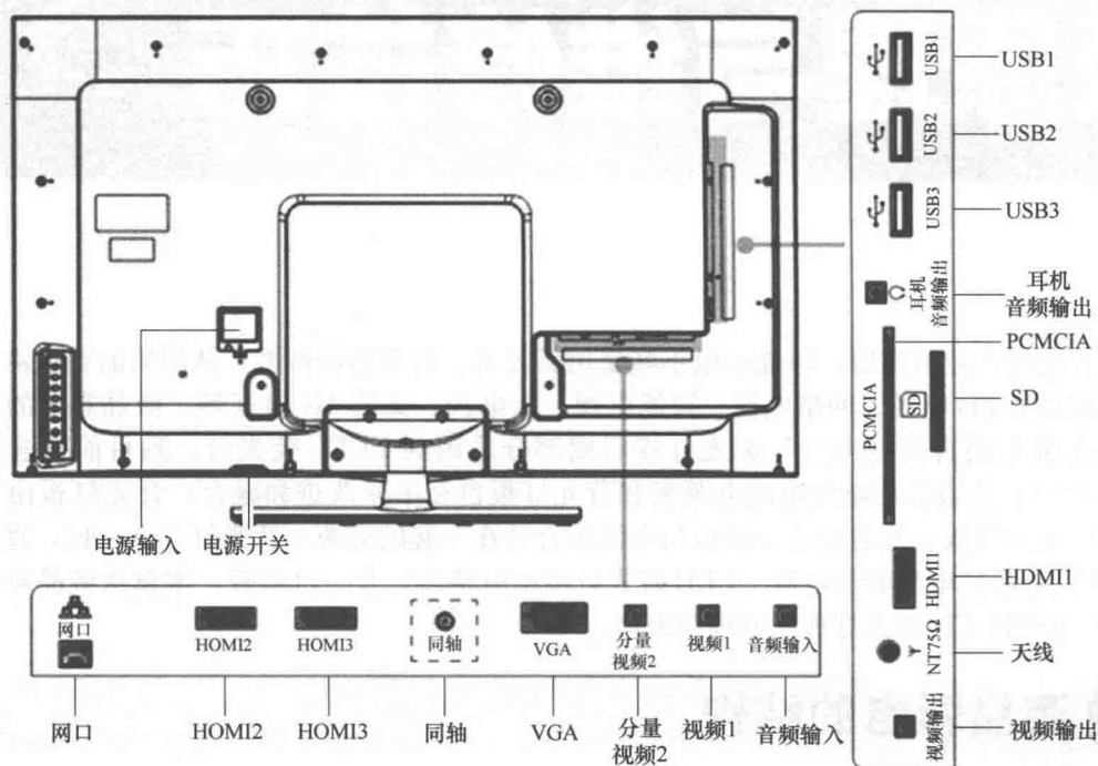
图 1-2 液晶电视机的背面
