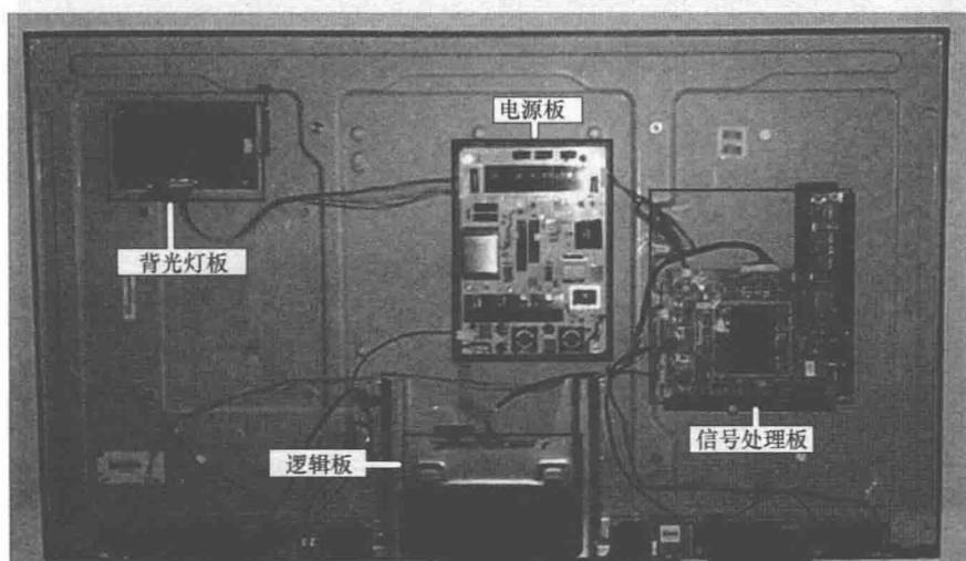
图 1-4 LED 液晶彩电电路组成
