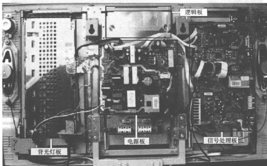
图 1-3 早期 LCD 液晶彩电电路组成
