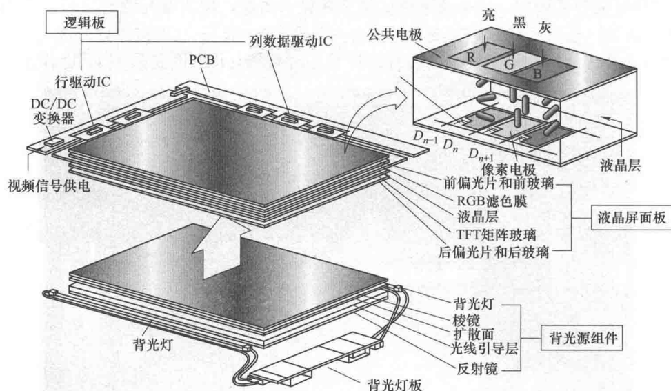
图 1-10 液晶屏组件结构图
