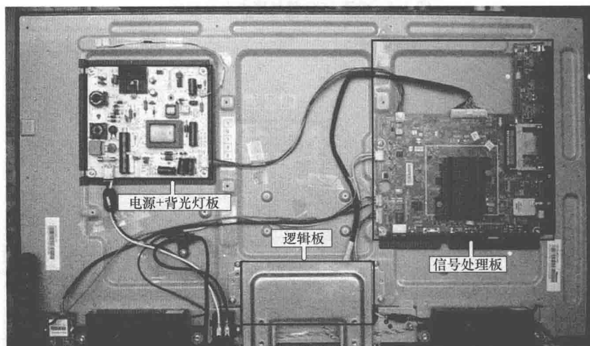
图 1-6 采用二合一板的 LED 液晶彩电电路组成
