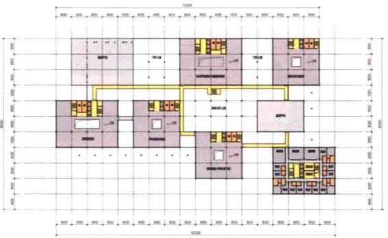
三层平面图 FLOOR PLAN 2
