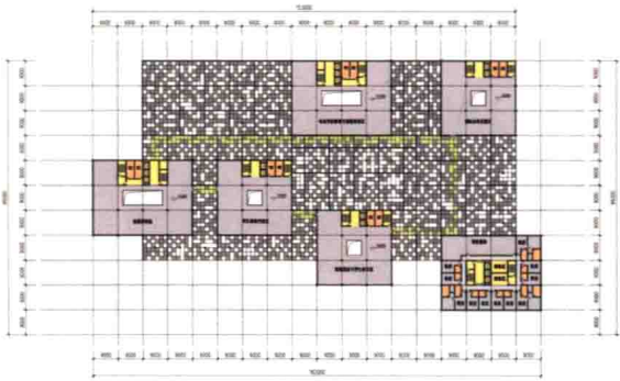
四层平面图 FLOOR PLAN 3
