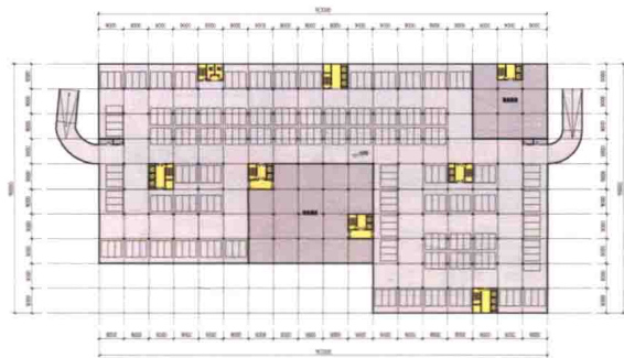
五层平面图 FLOOR PLAN 4
