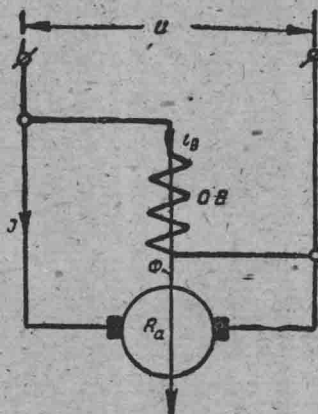
图 2—2 並激电动机的线路图
