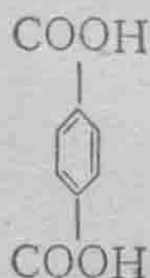
对-苯二甲酸
