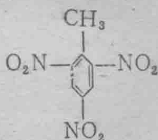
2, 4, 6-三硝基甲苯
