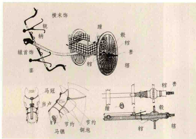
▲ 车马器具临摹复原图及各部分名称
