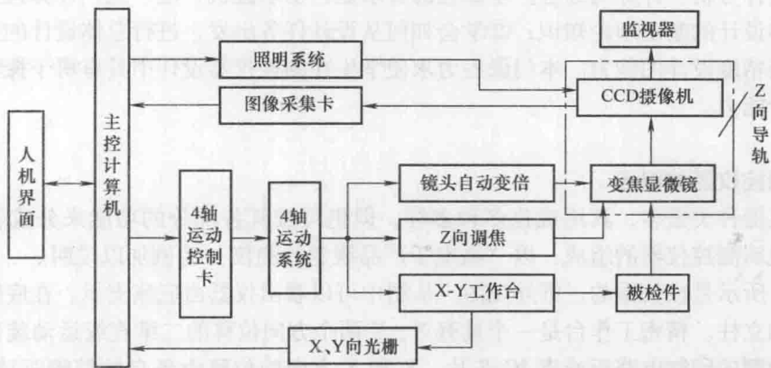
图 1-2 微电子产品视觉检测仪组成框图
