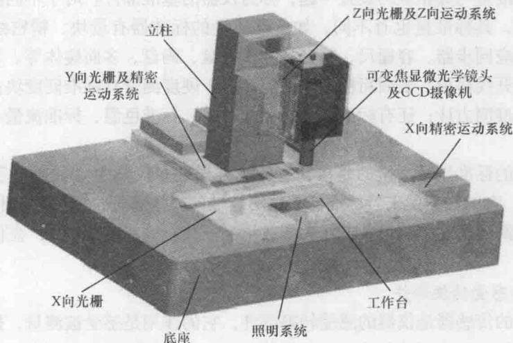
图 1-1 微电子产品视觉检测仪外观图
