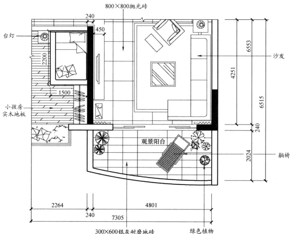
图 1-4 某室内装饰平面图 (四)
