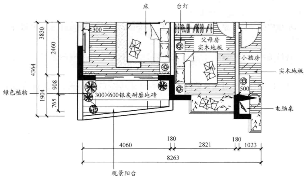
图 1-3 某室内装饰平面图 (三)
