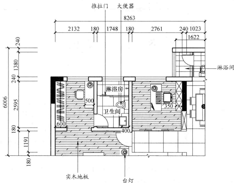
图 1-1 某室内装饰平面图（一）
