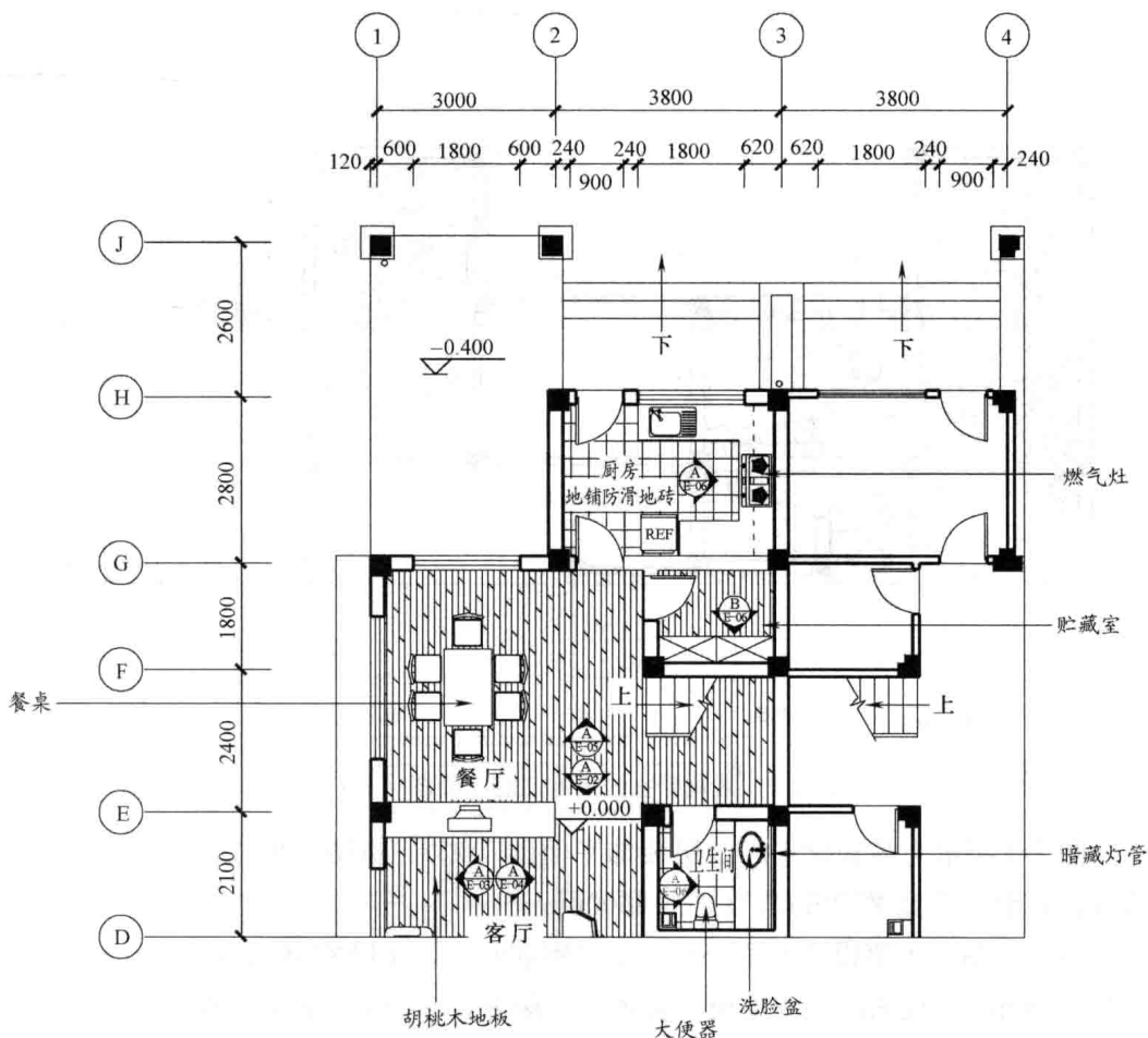
图 2-1 某别墅室内装饰一层平面图(一)
