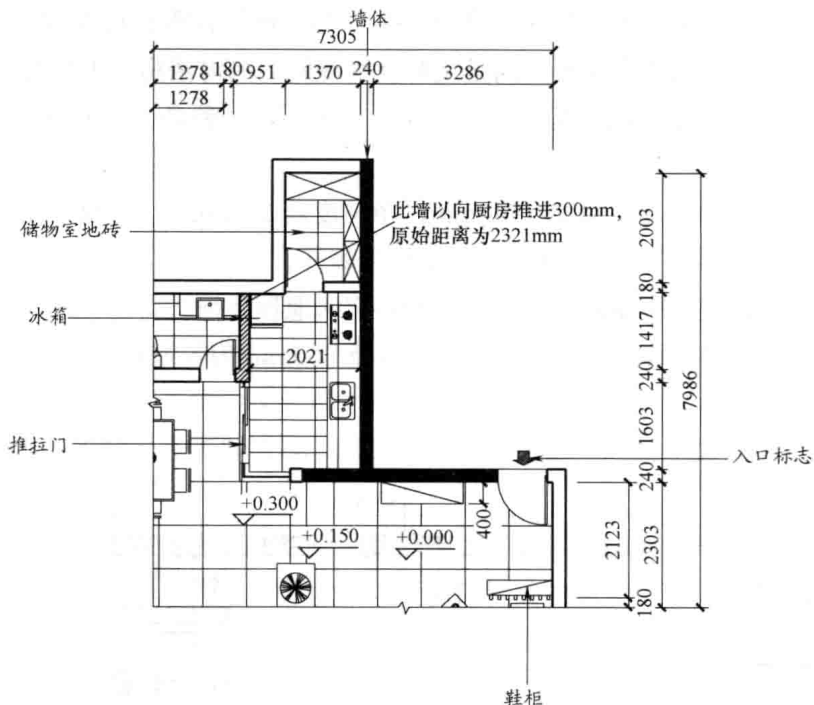
图 1-2 某室内装饰平面图（二）
