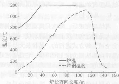
图 2.2 典型奥氏体不锈钢退火工艺曲线
