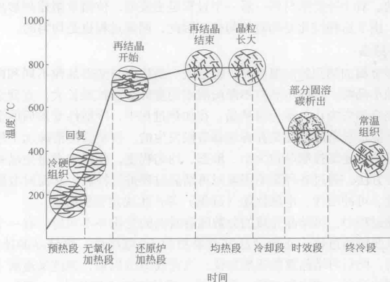
图 2.3 带钢在退火炉内再结晶过程示意图
