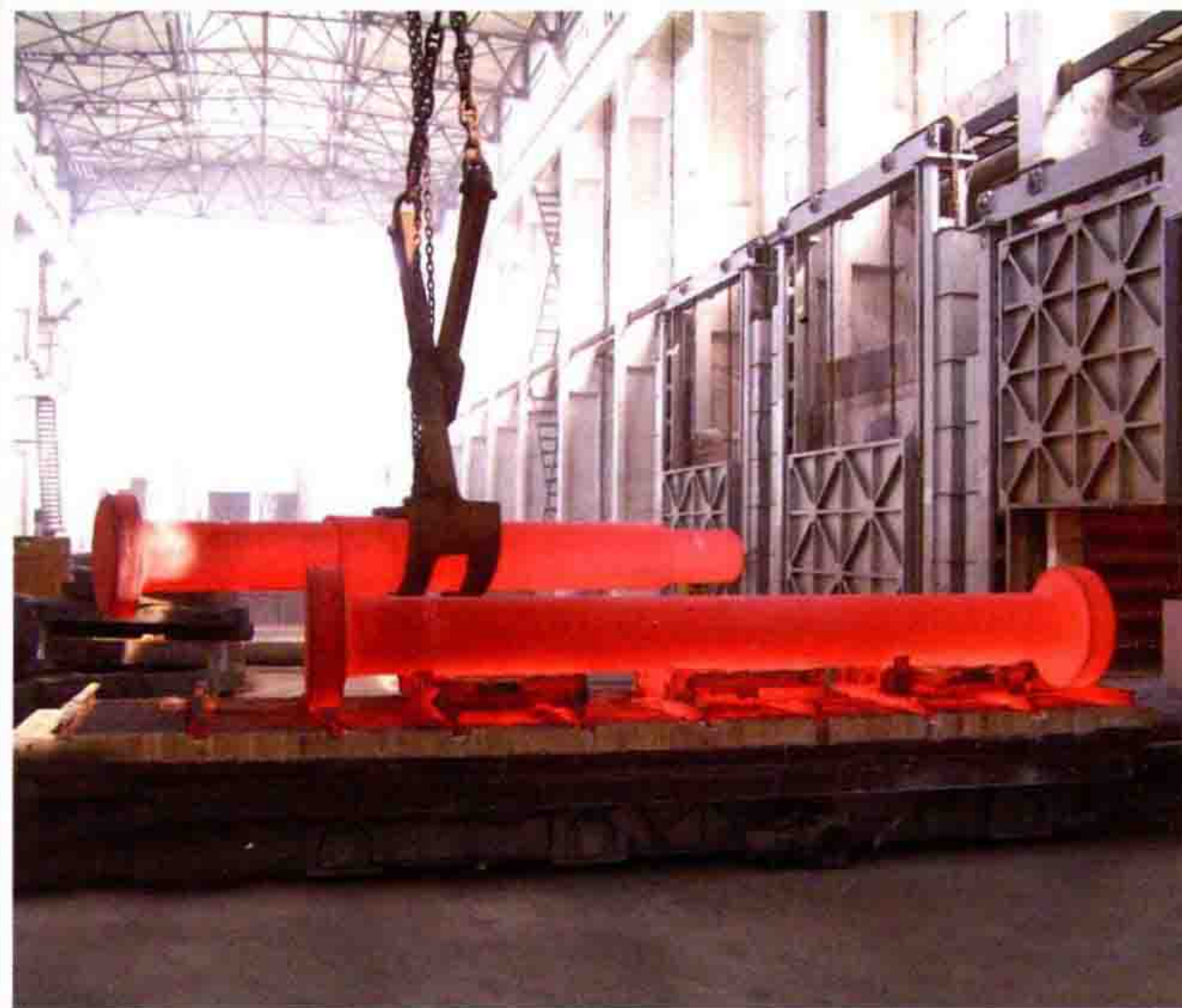
出炉工件
