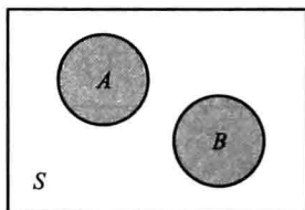
图 1-5 A \cap B = \emptyset
