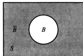
图 1-6 B 与 \bar{B}
