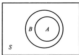
图 1-1 A \subseteq B
