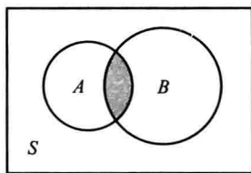
图 1-2 A \cap B
