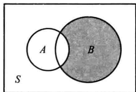
图 1-4 B - A
