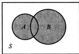
图 1-3 A \cup B
