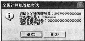
图1.3 信息验证
