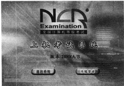
图1.1 登录界面
