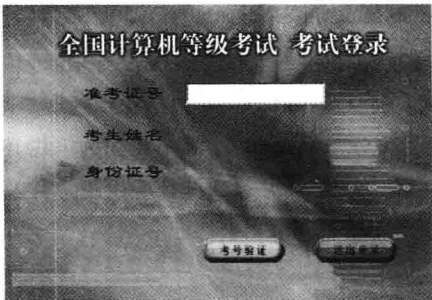
图1.2 身份验证
