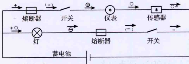
线路符号表达示意简图
