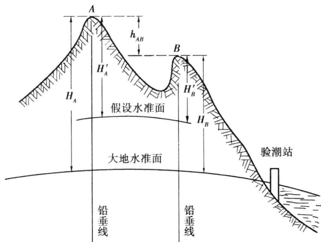
图 1.8 高程和高差
