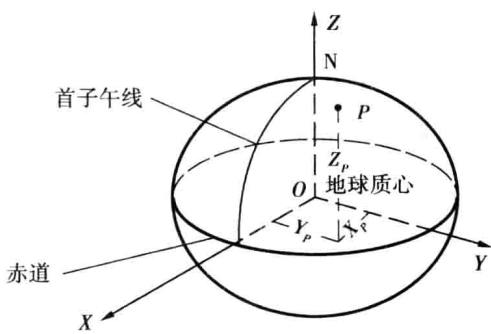
图 1.9 空间直角坐标系
