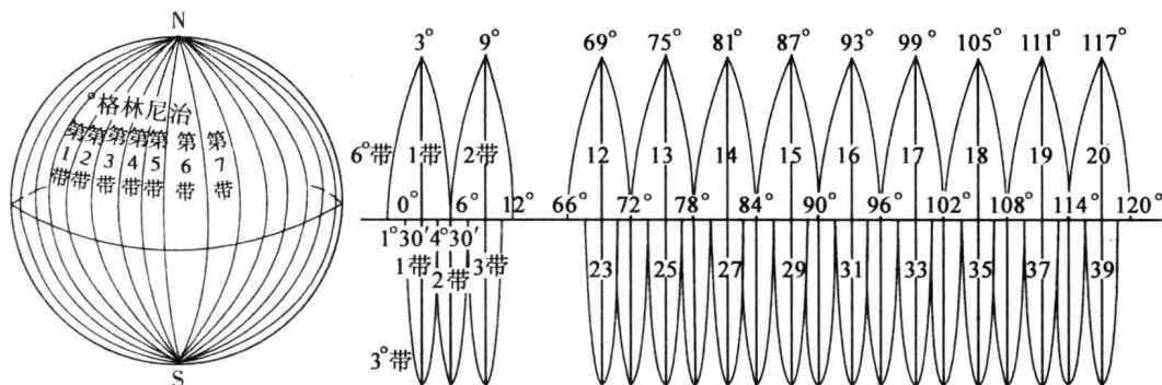
图 1.5 6^\circ 带和 3^\circ 带投影
