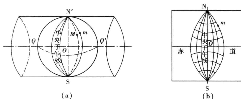
图 1.4 高斯投影
