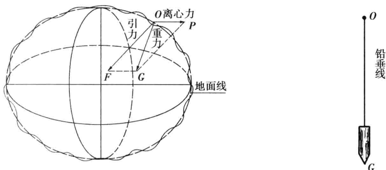
图 1.1 地球重力线
