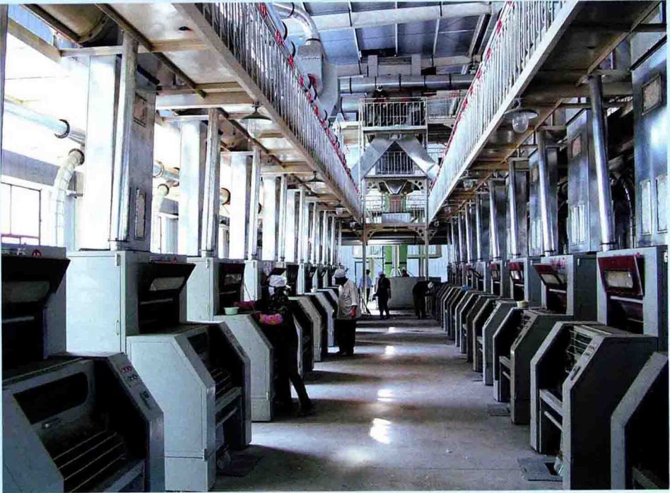
棉花加工生产线
