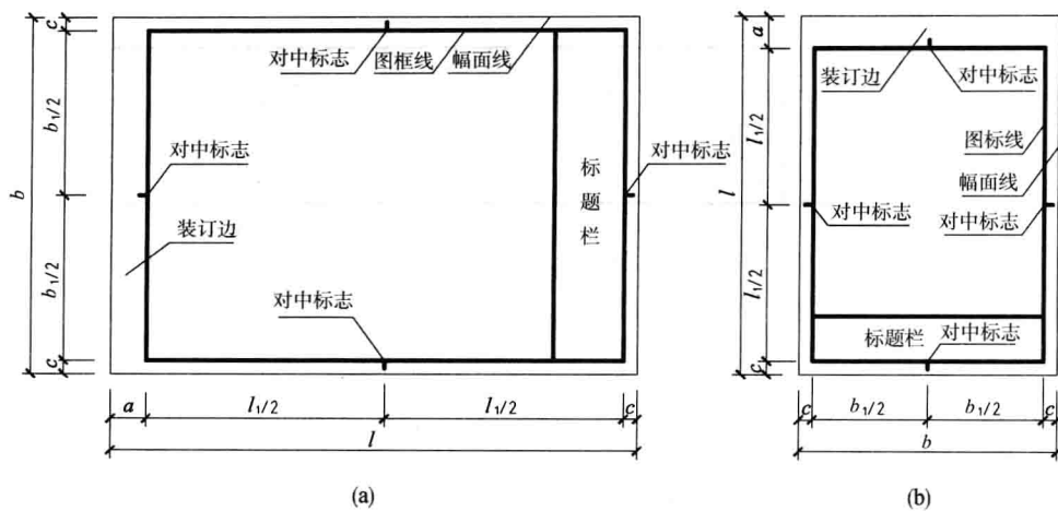
图 1-1 幅面代号的意义
