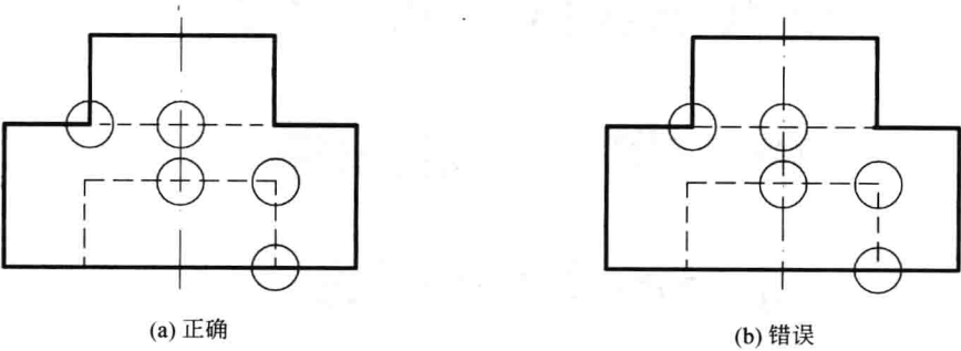
图 1-5 虚线交接的画法
