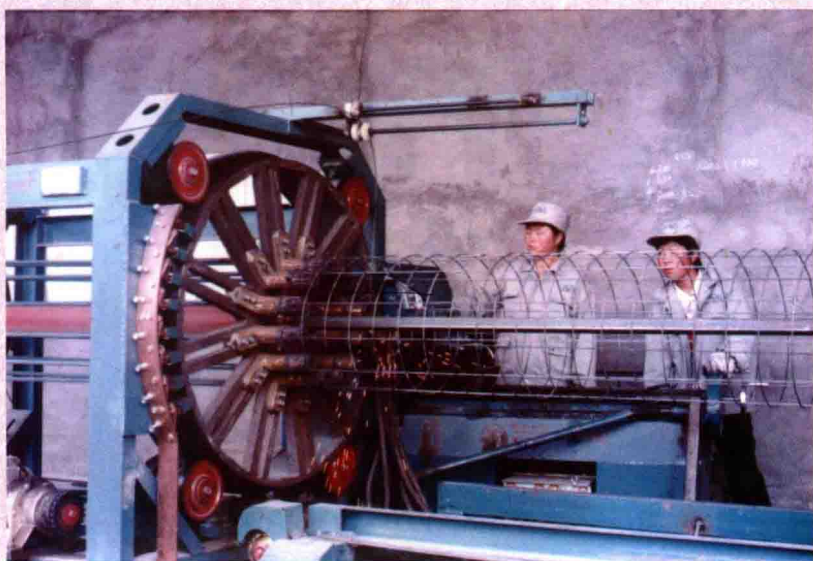
加工涵管盘骨
