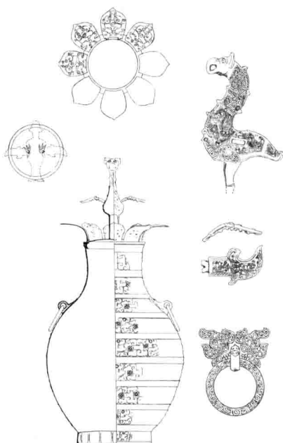
圖四 八瓣鳳鳥華蓋壺（山彪鎮一號墓）
