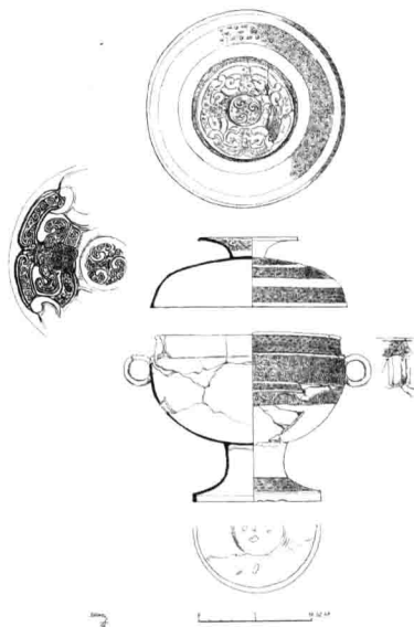
圖五 帶蓋雙環豆（山彪鎮一號墓）
