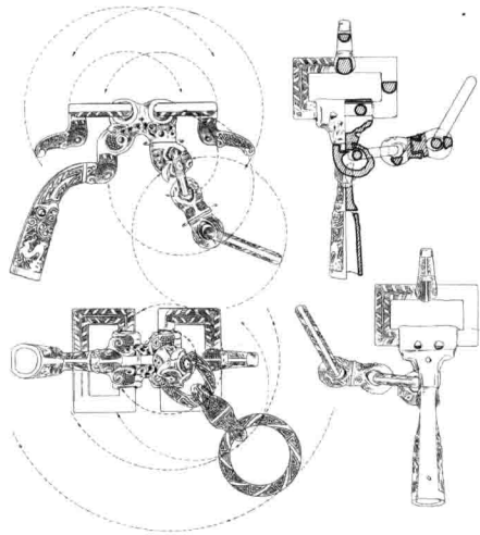
圖六 活動卡環（山彪鎮一號墓）
