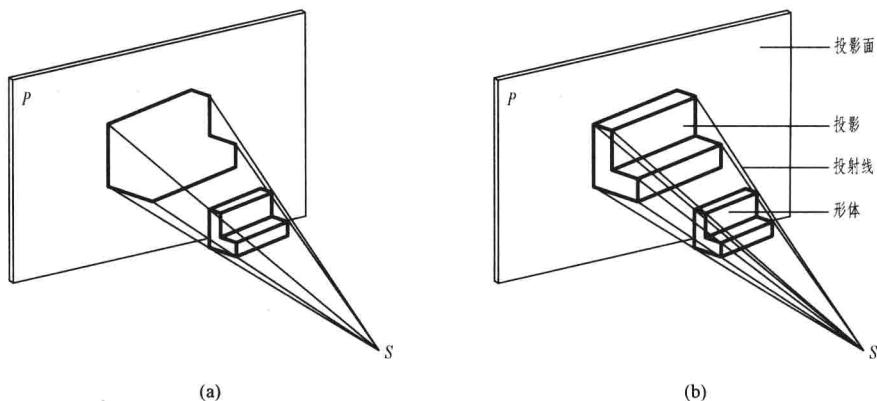
图 1-1-2 形体的投影
