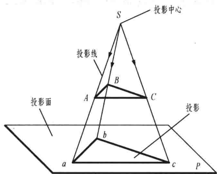
图 1-1-1 中心投影法
