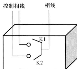
图 1-1-5 开关接线图
