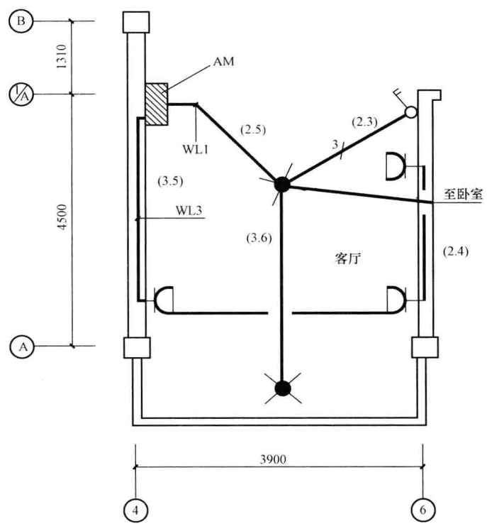
图 1-1-2 某住宅楼客厅局部照明平面图
