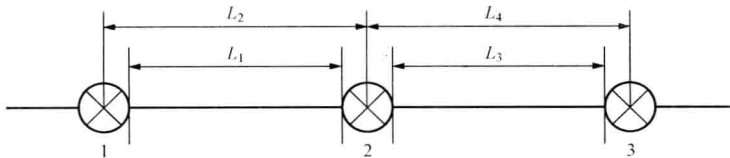
图 1-1-6 电气配管延长米的计算
