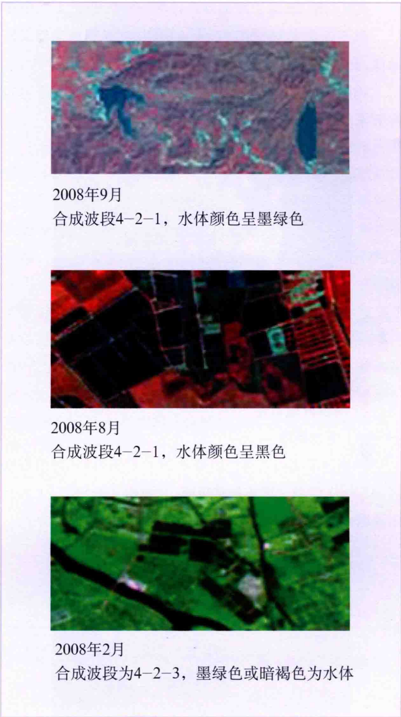
图 1-3-2 不同波段合成图
