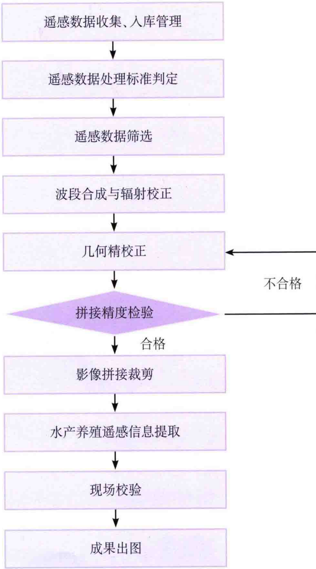
图 1-3-1 水产养殖水体资源遥感普查技术流程图
