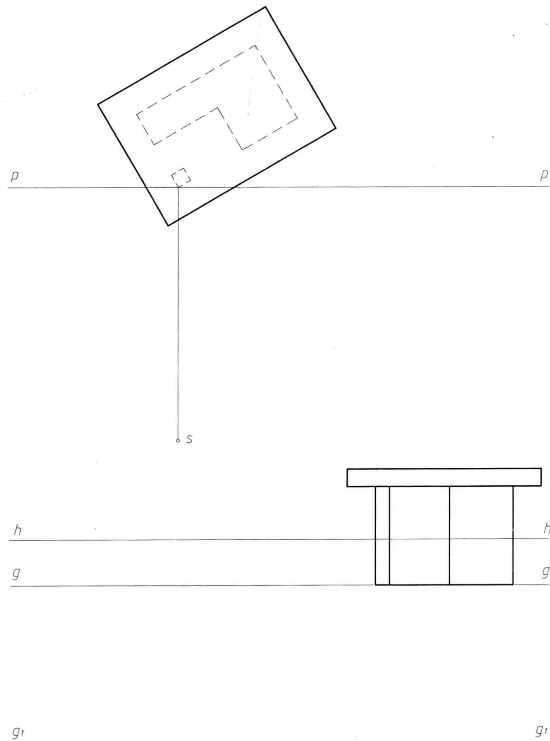
2-8 用迹点灭点法作建筑形体的两点透视(要求先降低基线作透视平面图)。
