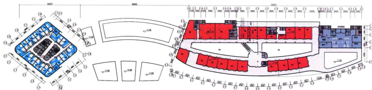
三层平面图
