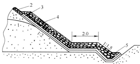
图 2F311012-3 贴坡排水
