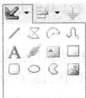
图 1.1.11 绘图子菜单
