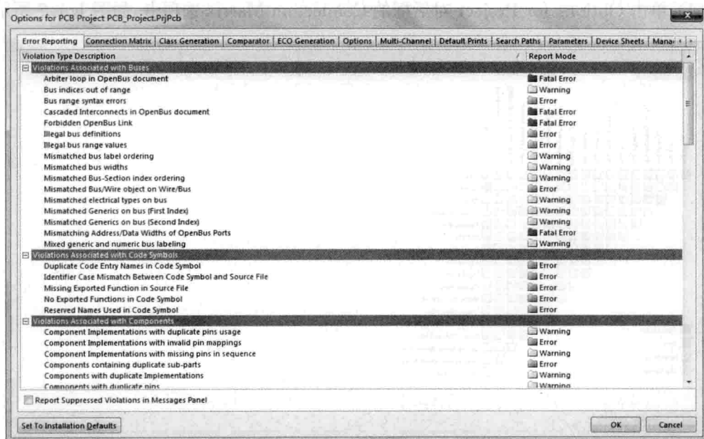
图 1.1.6 Options for Project 对话框
