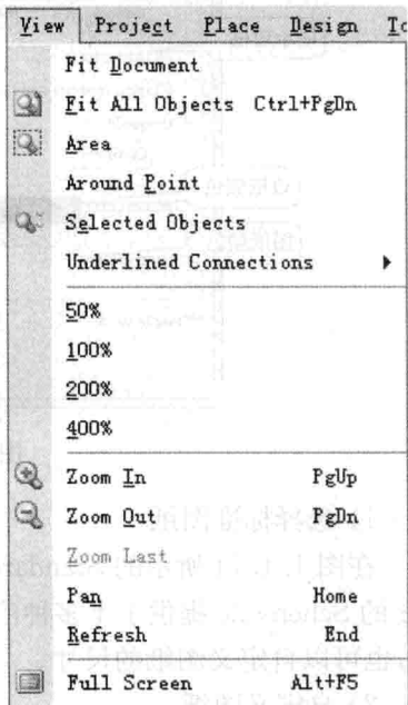
图 1.1.13 View 菜单
