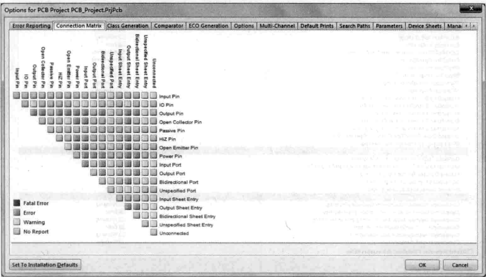
图 1.1.7 Connection Matrix 选项卡
