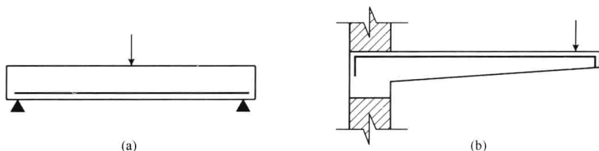
图 1-2 受拉钢筋在构件中的位置 (a)简支梁；(b)雨篷
