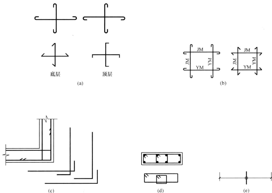
图 1-10 钢筋常见画法
