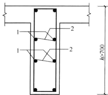
图 1-8 腰筋与拉筋布置
