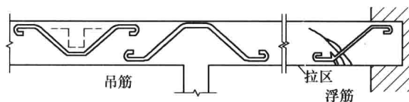
图 1-5 吊筋布置图
