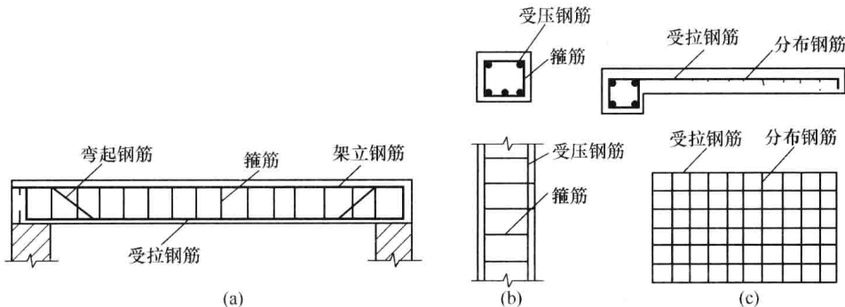
图 1-1 钢筋在构件中的种类 (a)梁;(b)柱;(c)悬臂板
