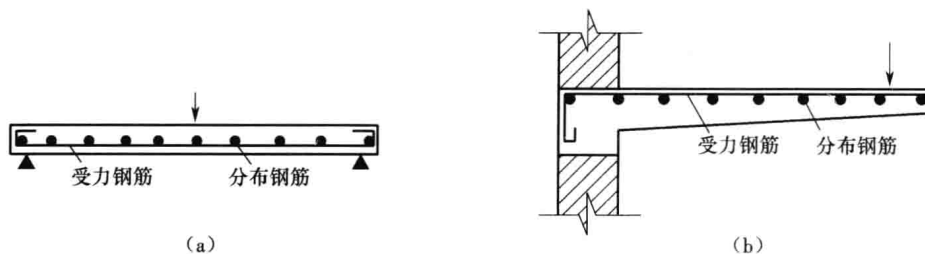
图 1-7 分布钢筋在构件中的位置
