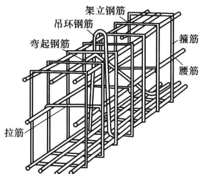
图 1-6 架立筋、腰筋等在钢筋骨架中的位置
