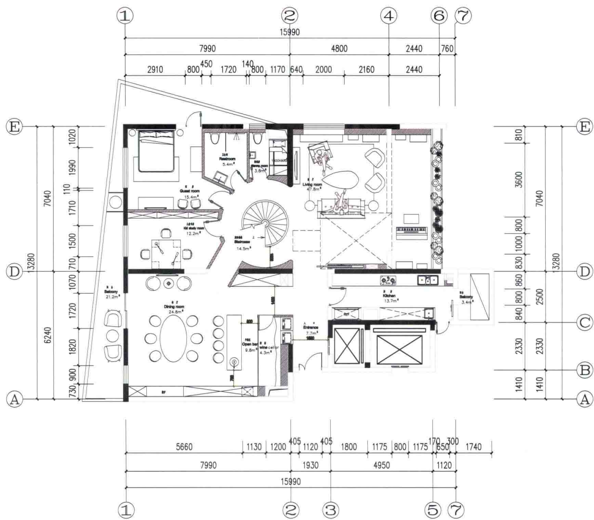
一层平面图
