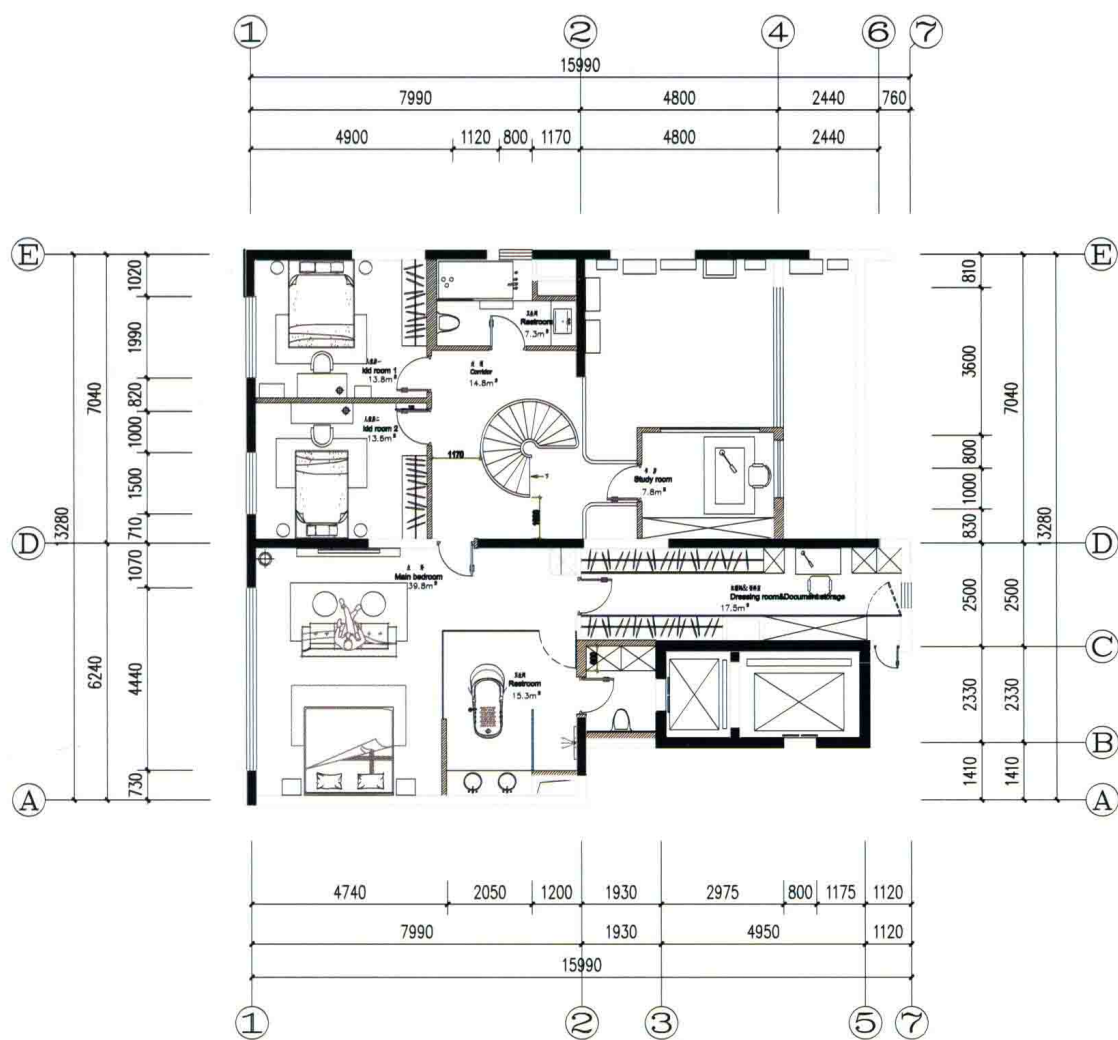
二层平面图
