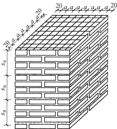
图 1. 1. 1 网状配筋砖柱
