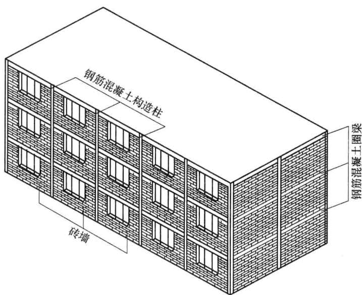
图 1.1.4 内嵌式组合砖墙
