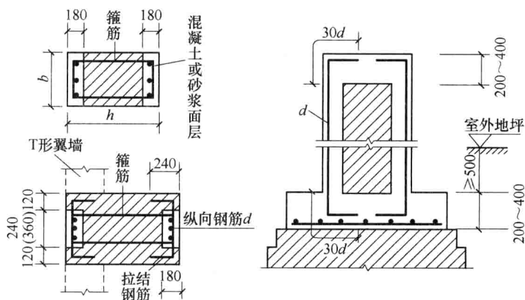
图 1.1.3 外包式组合砖柱
