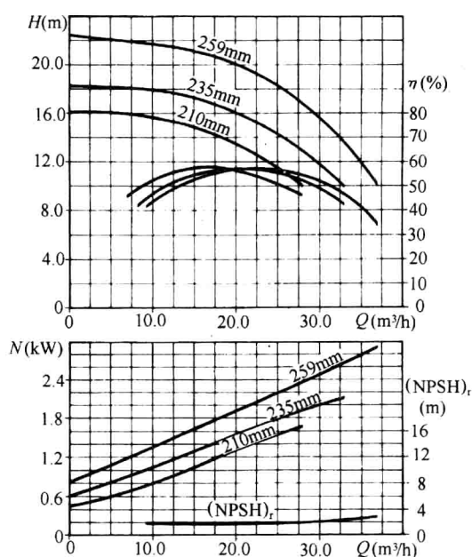
图 3-10 CM40-250 型泵性能曲线 ( n = 1450\text{r/min} ) ( DN65/40 )
