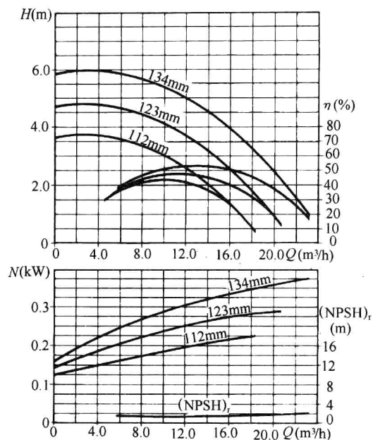
图 3-7 CM32-125 型泵性能曲线 ( n = 1450\text{r/min} ) ( DN65/40 )
