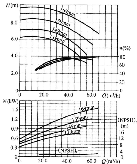
图 3-16 CM65-160 型泵性能曲线 ( n = 1450 \text{ r/min} ) ( DN80/65 )
