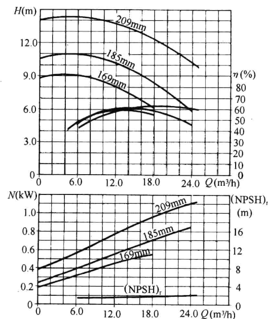
图 3-9 CM40-200 型泵性能曲线 ( n = 1450\text{r/min} ) ( DN65/40 )
