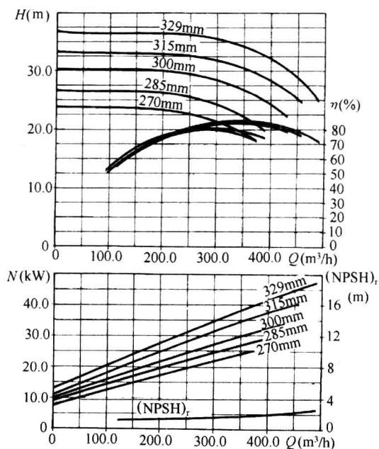
图 3-31 CM150-315 型泵性能曲线 ( n = 1450 \text{ r/min} ) ( DN200/150 )
