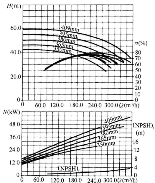
图 3-30 CM125-400 型泵性能曲线 ( n = 1450 \text{ r/min} ) ( DN150/125 )
