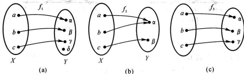
图 1-3 单射、满射与双射
