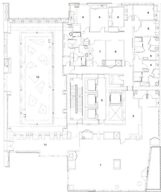
底层平面图
