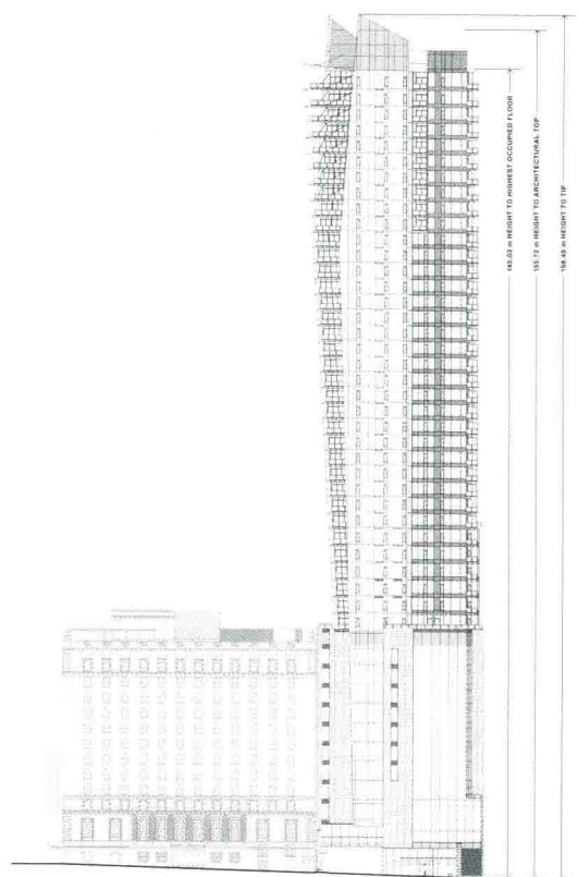
东立面图
