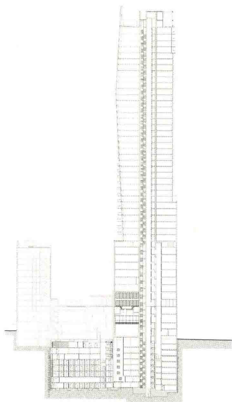
剖面图
