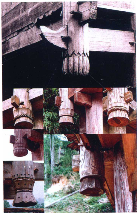
图3 吊柱花饰之一
