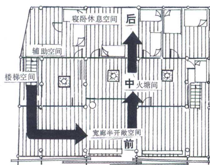
图5 侗居平面空间序列图
