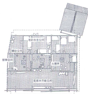
图4 侗居基本平面图
