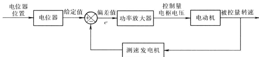
图 1-7 电动机转速闭环控制方框图
