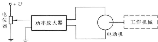
图 1-4 直流电动机转速开环控制系统
