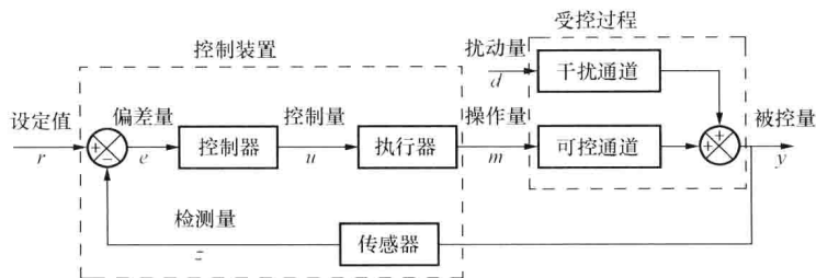
图 1-3 反馈控制系统方框图
