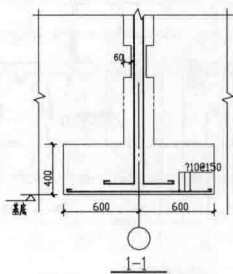
图 1-11 基础详图
