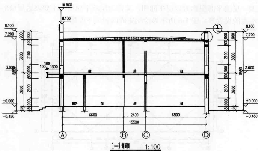
图 1-8 建筑剖面图
