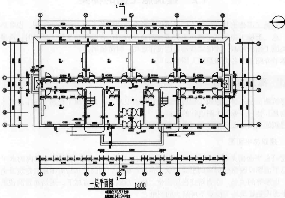
图 1-4 一层平面图
