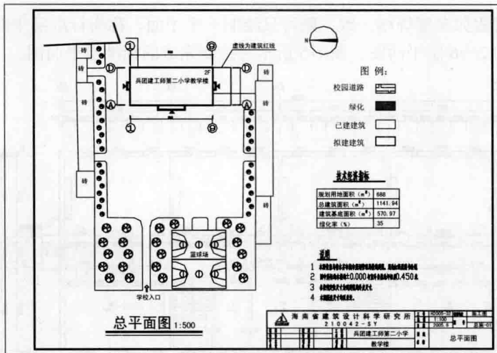
图 1-3 建筑总平面图
