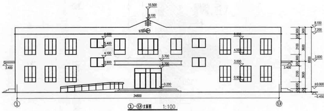
图 1-7 建筑立面图
