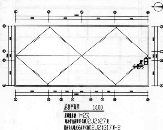
图 1-6 屋顶平面图
