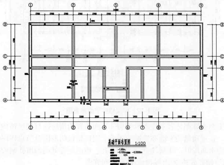
图 1-10 基础平面图
