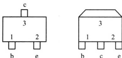
图 2-7 常见三极管引脚排列
