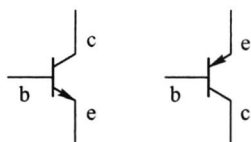
图 2-5 三极管的符号
