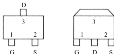
图 2-8 常见场效应管引脚排列
