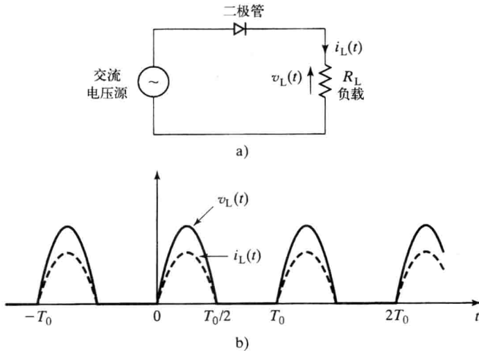
图 1-12 半波整流器
