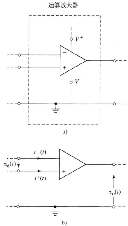
图 1-5 运算放大器
