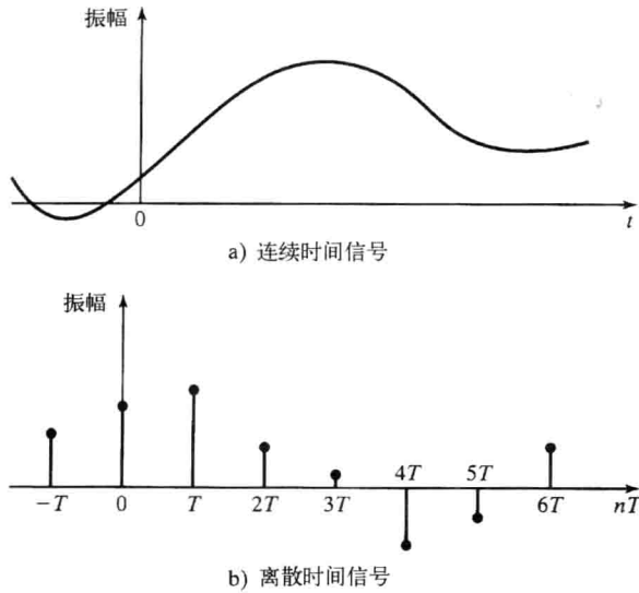
图 1-2 信号
