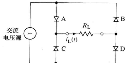
图 1-14 全波整流器
