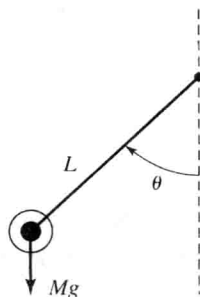
图 1-9 单摆
