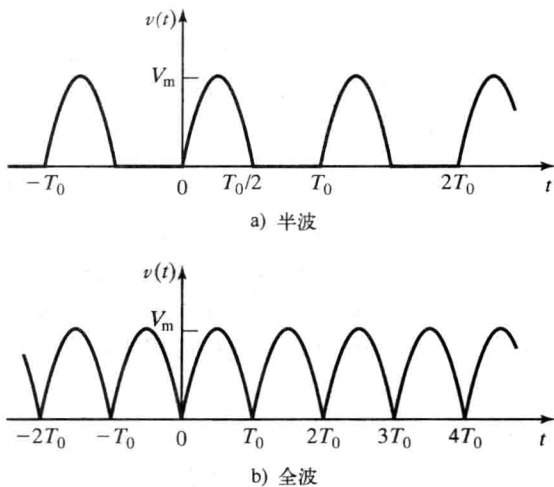
图 1-10 整流信号
