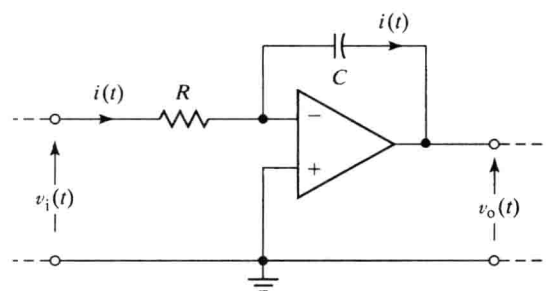
图 1-7 积分放大器
