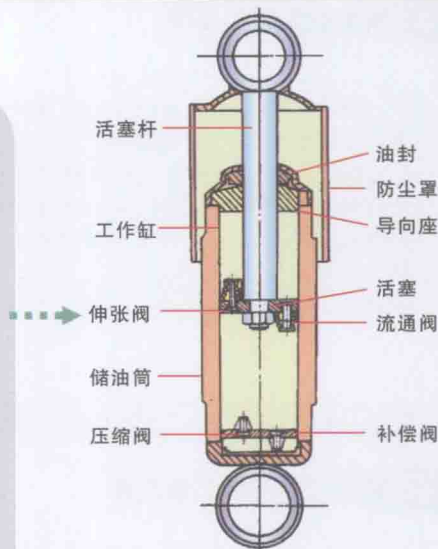
双向作用筒式减振器
