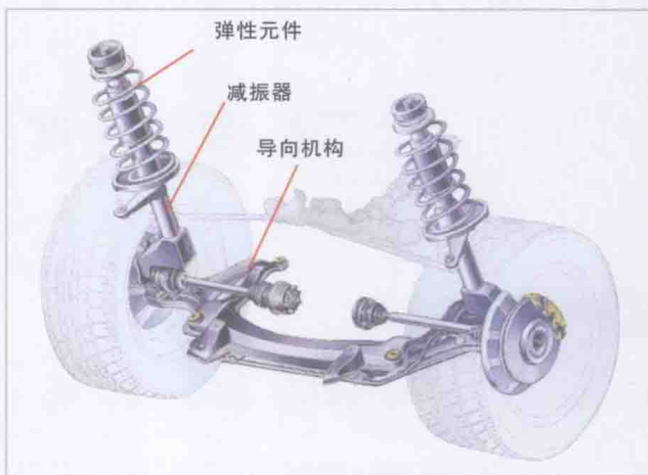
悬架系统组成图
