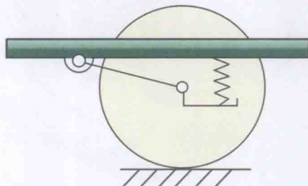
纵臂式独立悬架
