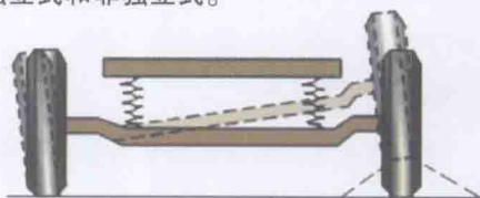
非独立式悬架
