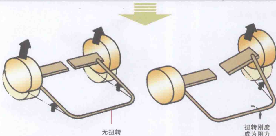
横向稳定杆工作示意图
