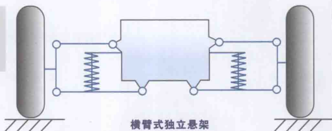
横臂式独立悬架
