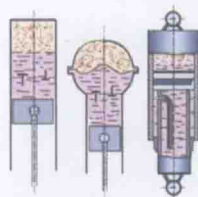
油气弹簧
