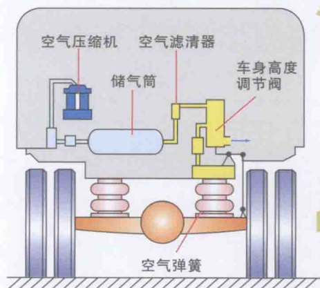
空气弹簧式非独立悬架结构示意图
