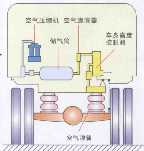
空气弹簧式非独立悬架
