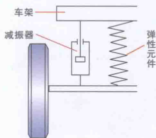
减振器和弹性元件安装方式
